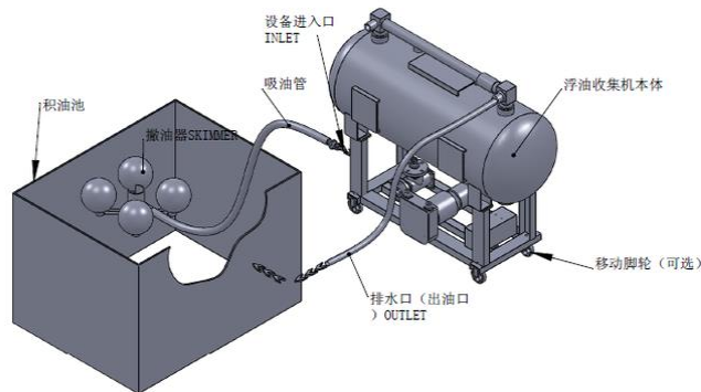
图 16 浮油设备图
