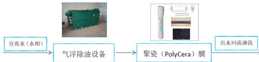
图 15 含油污水处理工艺流程
