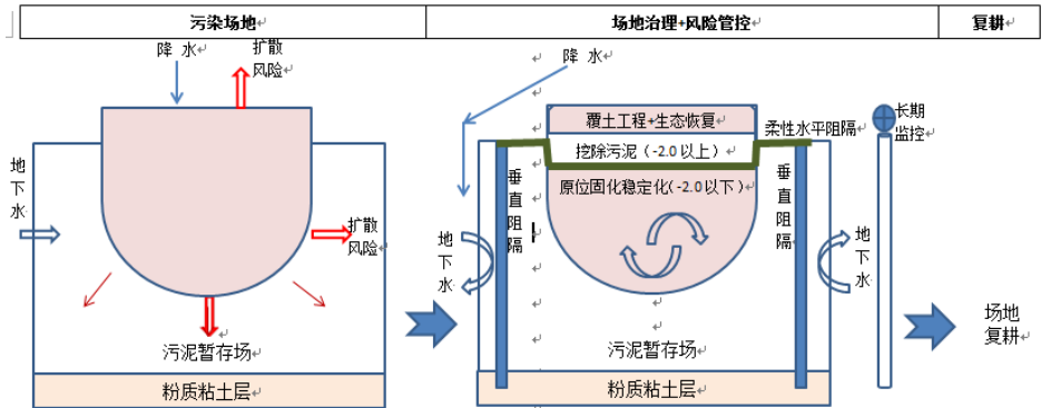
图 8 修复工艺
