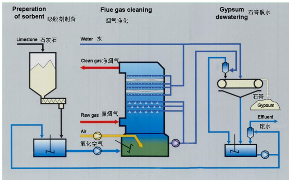
图 14 烟气脱硫工艺流程
