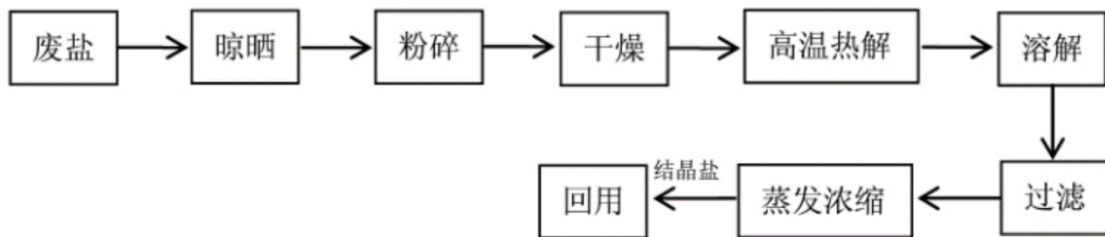
图 19 微波热解工业盐工艺流程
