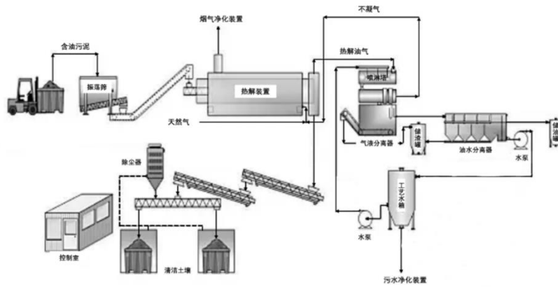
图 10 油土处理处置工艺流程图
