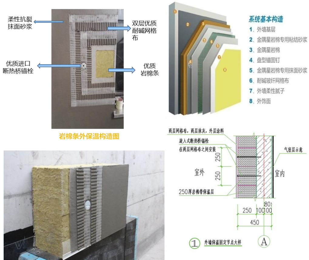
图 4 建筑保温材料
