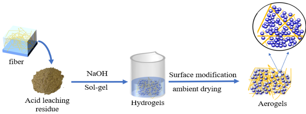
图 3 气凝胶制备流程
