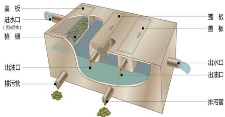
图 11 油水分离器加盖板封闭回收 VOCs
