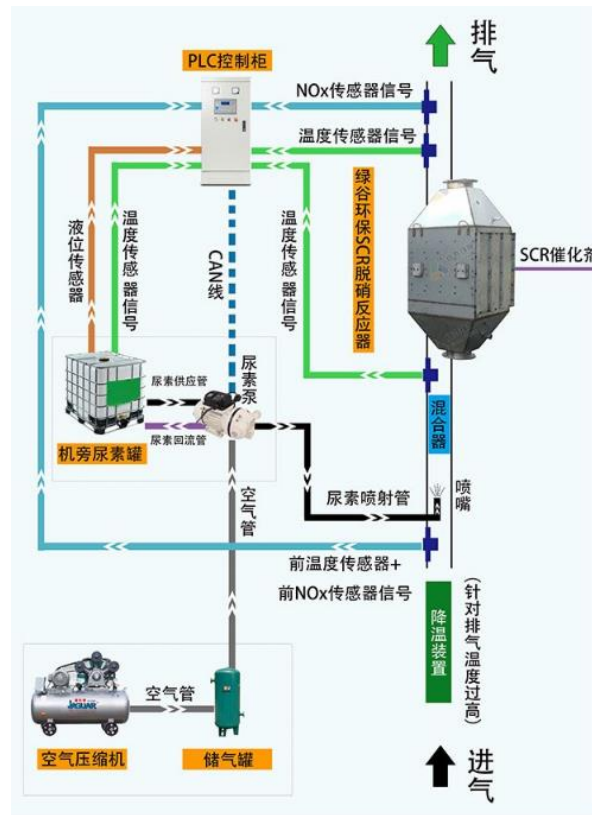
图 13 SCR 烟气脱硝系统
