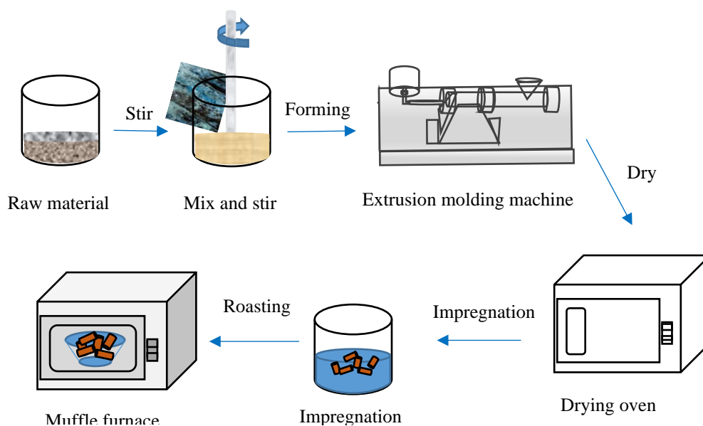
图 1 粉煤灰催化剂制备流程
